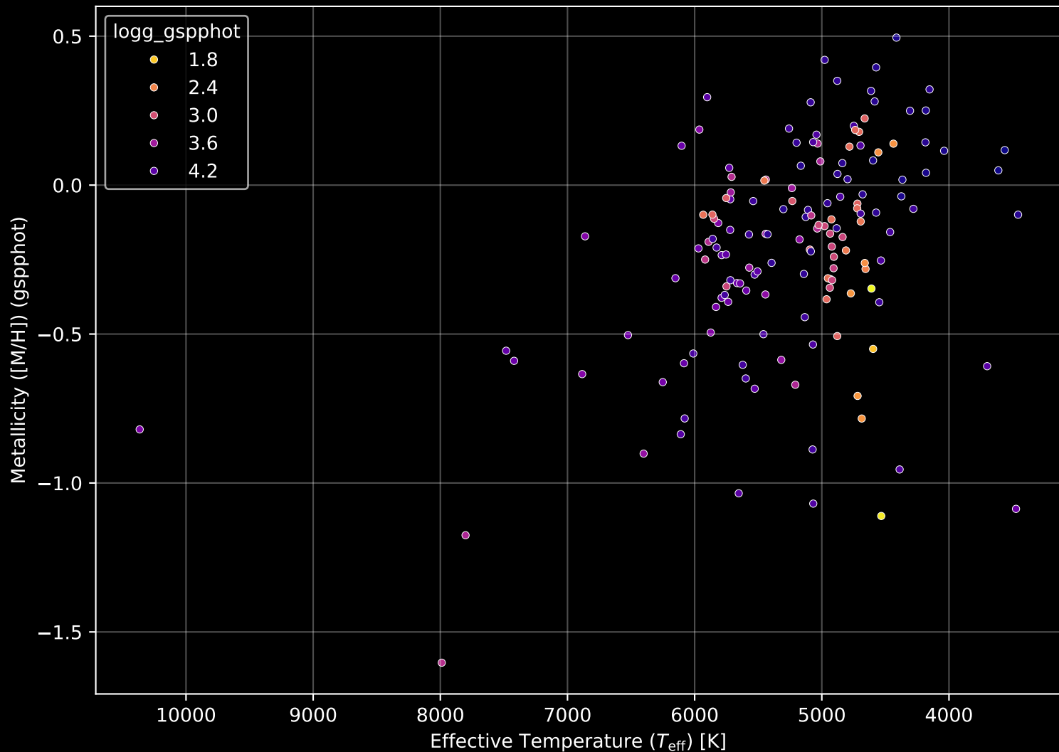
APOGEE DR17 Field: [060-30] Stellar Population Parameters (n= 154)
